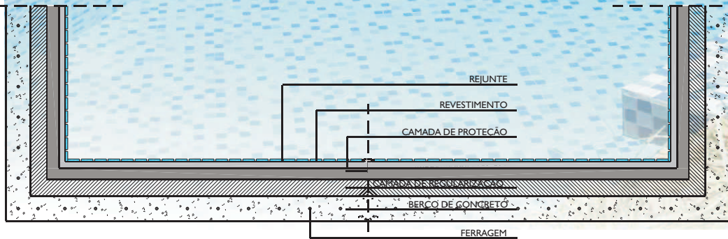
CORTE ESQUEMÁTICO - IMPERMEABILIZAÇÃO PISCINA
